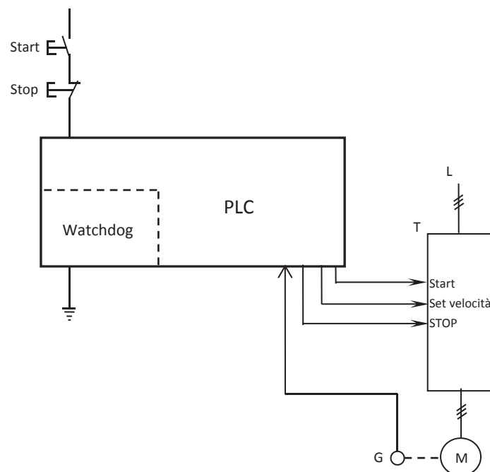
Fig. 36: Schema circuitale
