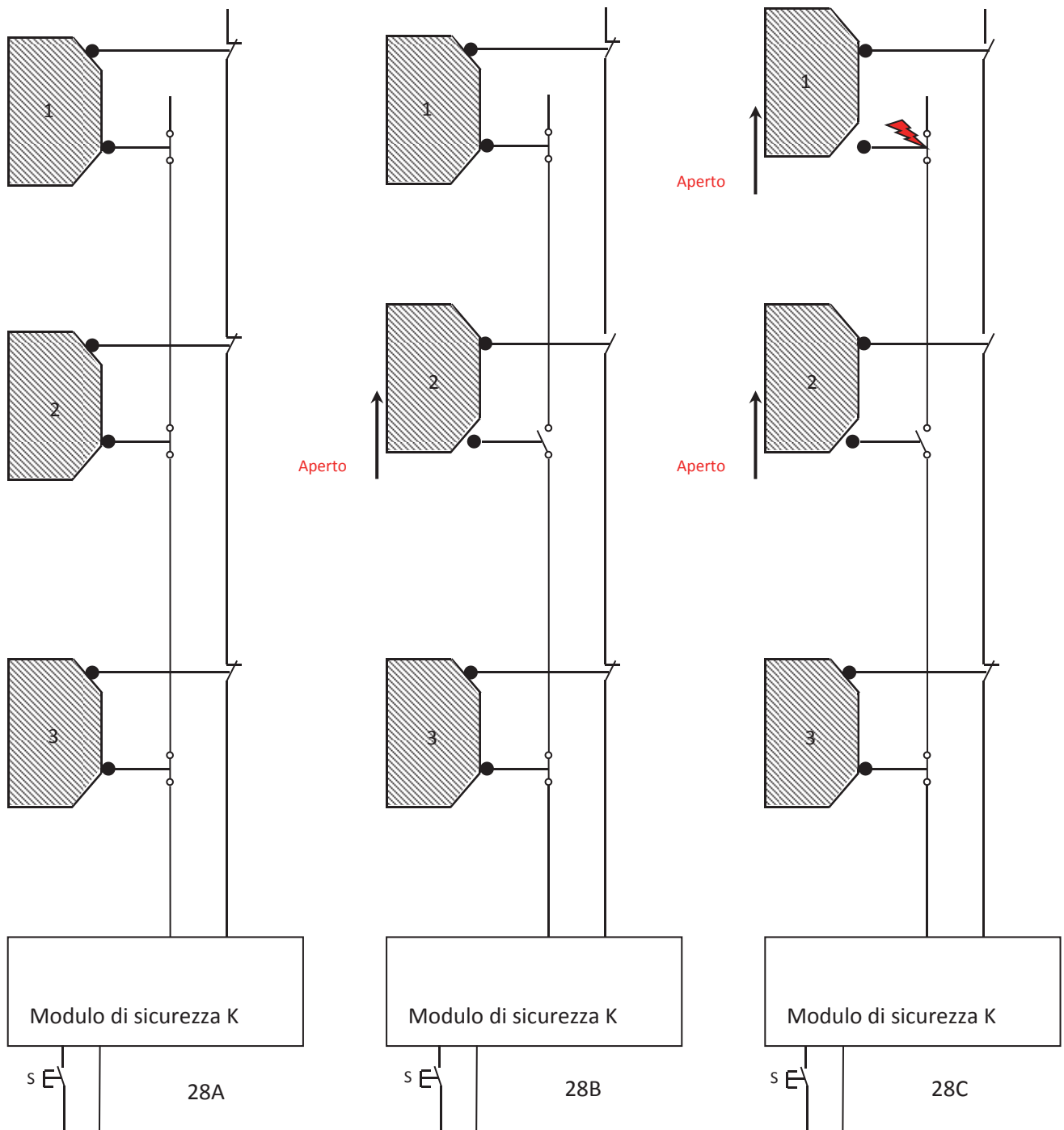
Figg. 28A, 28B, 28C: Mascheramento diretto del guasto
