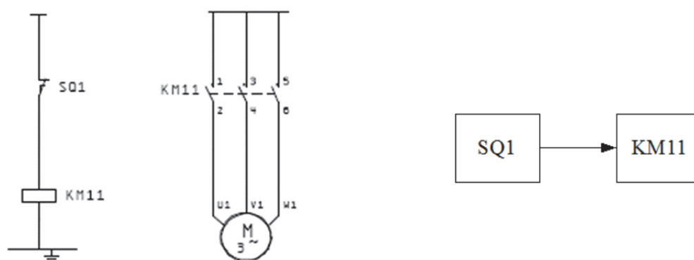
Fig. 31: Schema circuitale e diagramma a blocchi
