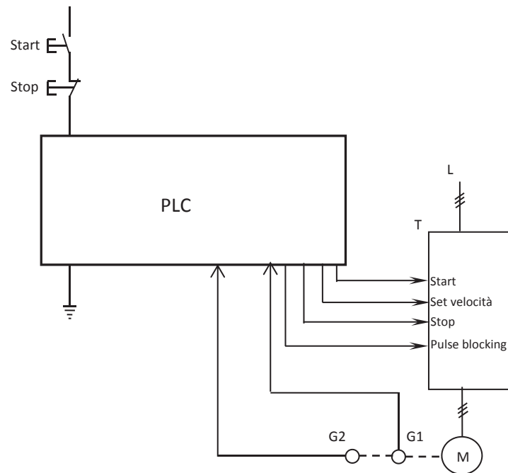
Fig. 39: Schema circuitale
